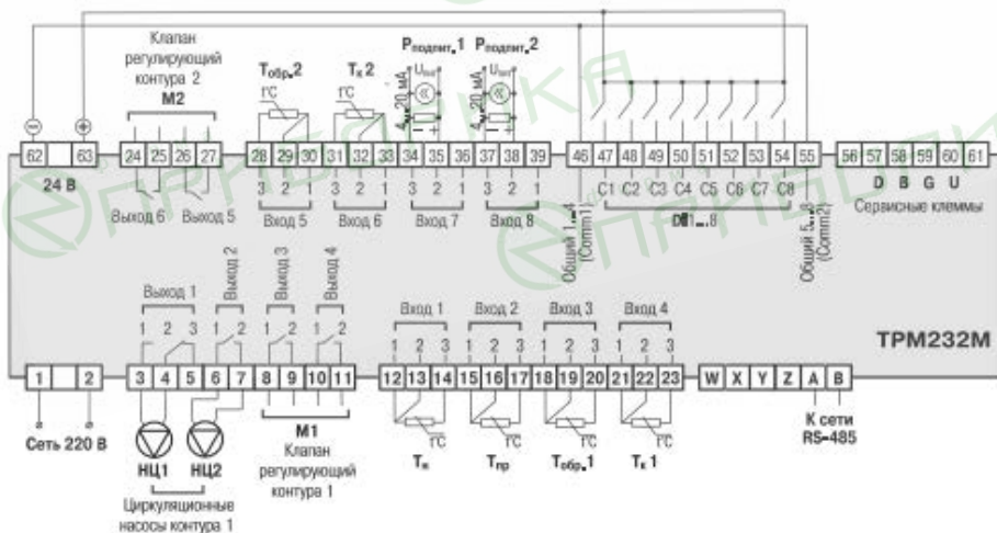
Схема 3. ПОДКЛЮЧЕНИЯ
