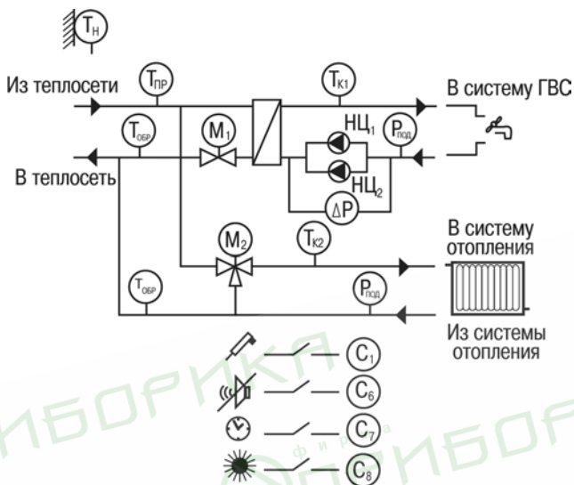
Схема 3. ПОДКЛЮЧЕНИЯ
