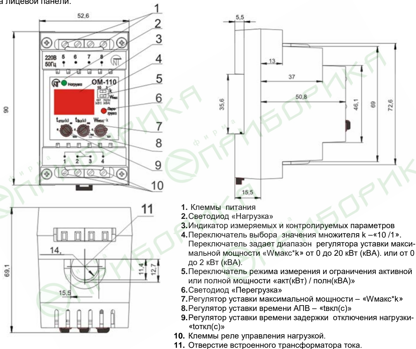
Рисунок 1- Внешний вид ОМ-110
