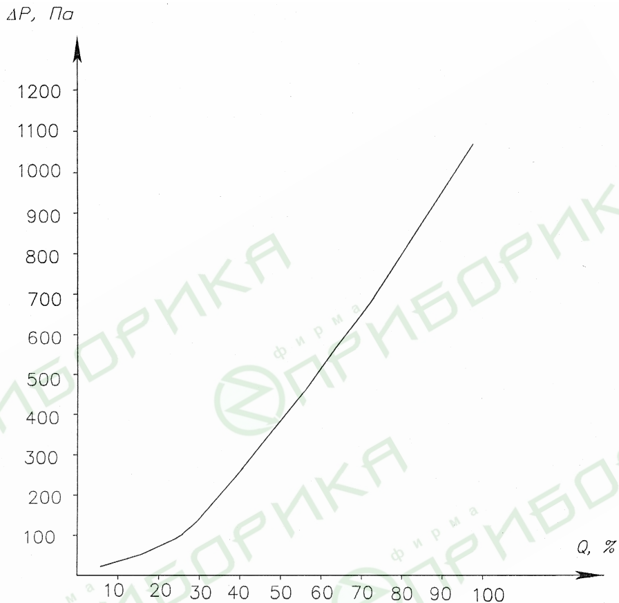
График зависимости потери давления на счетчике от расхода
