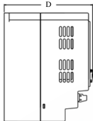
Рис. 1.5 Размеры преобразователей 1 ф, 220 В, 0,4 - 0,75 кВт
