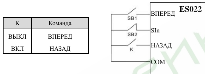
Рис. 6.12 Режим 3-проводного управления 1
