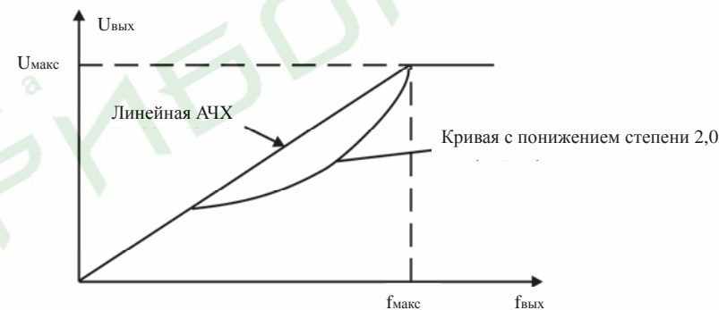
Рис. 6.8 Диаграммы АЧХ
