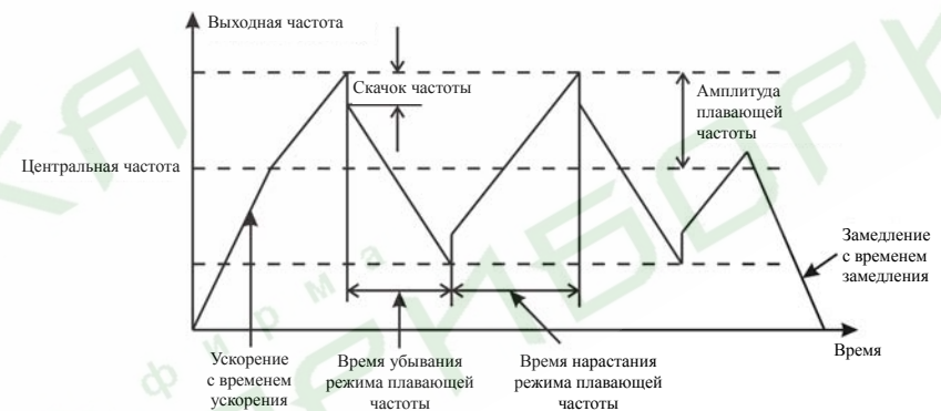
Рис. 6.17 Иллюстрация режима плавающей частоты
