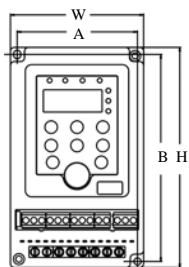
Рис. 1.5 Размеры преобразователей 1 ф, 220 В, 0,4 - 0,75 кВт
