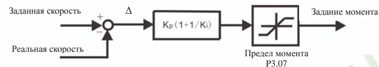
Рис. 6.6 Структура АРС
