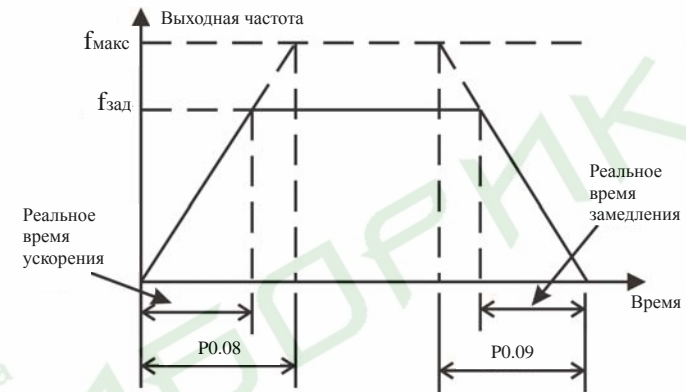
Рис. 6.1 Время ускорения и время замедления
