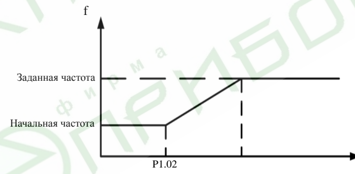
Рис. 6.3 Диаграмма запуска
