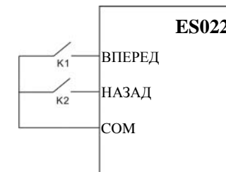
Рис. 6.11 Режим 2-проводного управления 2
