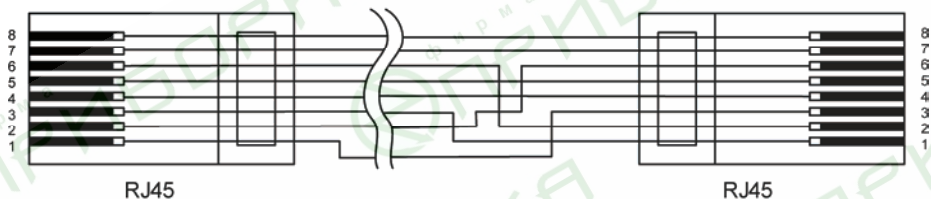
Рисунок Б.1 – Схема кабеля Ethernet Crossover
