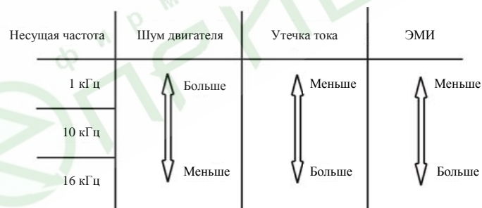
Рис. 6.3 Побочные явления при различных значениях несущей частоты ШИМ
