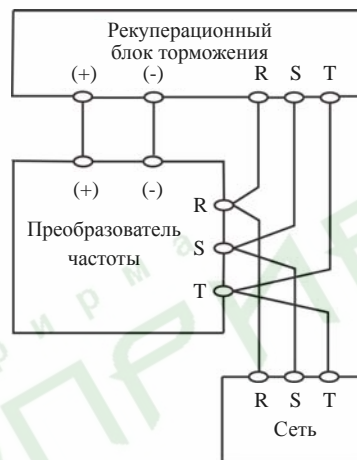
Рис. 4.11 Подключение рекуперационного блока торможения
