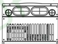
Рис. 1.6 Размеры преобразователей 18,5 - 110 кВт
