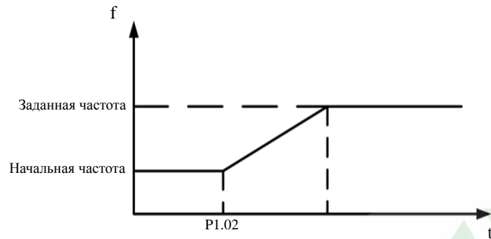
Рис. 6.4 Диаграмма запуска
