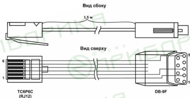
Рисунок Д.2 – Схема кабеля КС2
