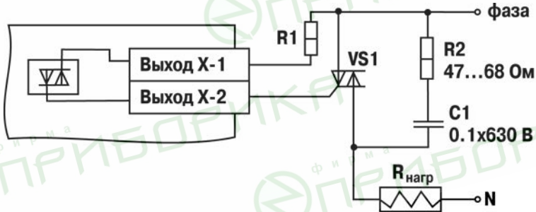
Рисунок Б.10 – Схема подключения нагрузки к ВУ типа С
