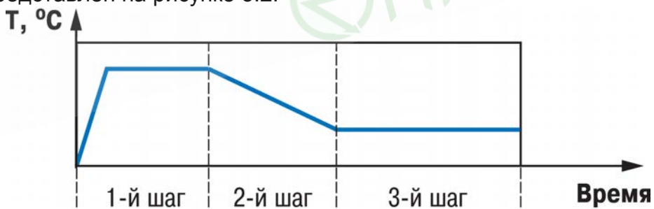
Рисунок 3.2 – Пример Программы технолога для ТРМ151
