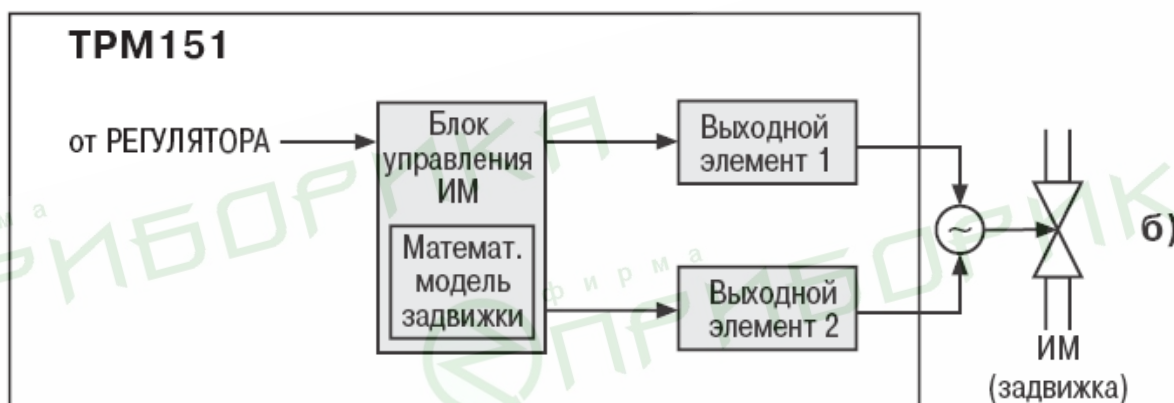
Рисунок 3.14 - Управление 3-х позиционным ИМ: а – с датчиком положения; б – без датчика приложения
