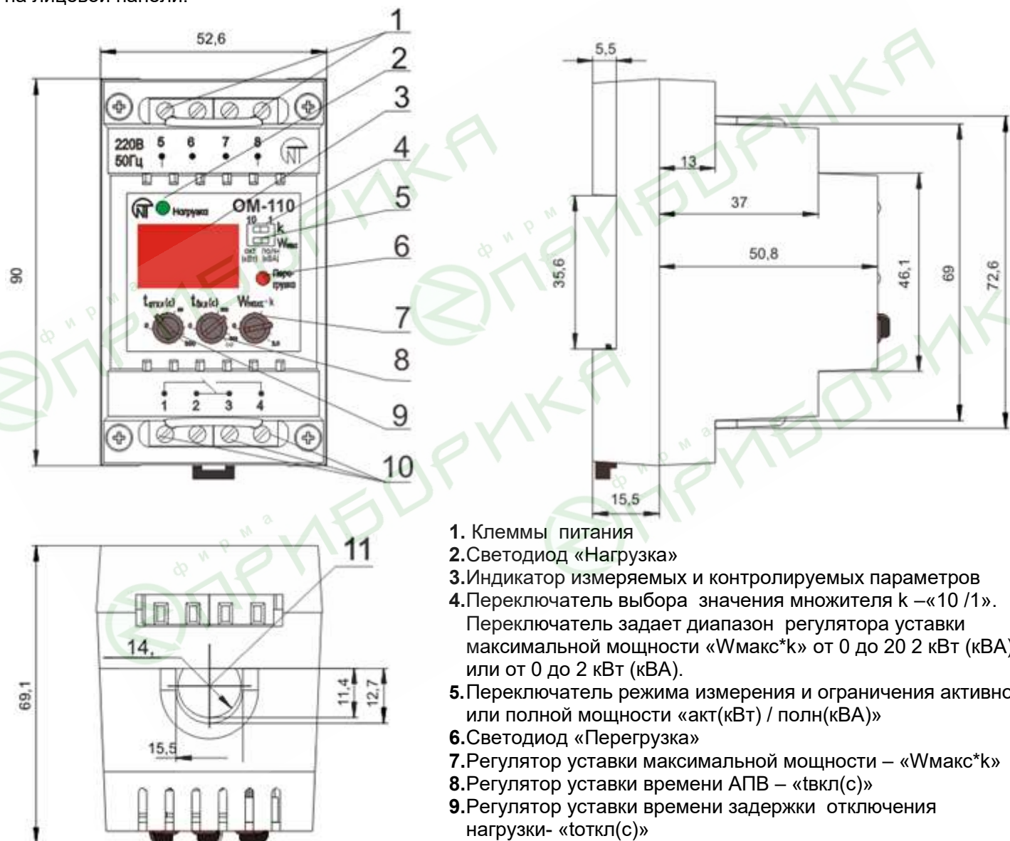
Рисунок 1- Внешний вид ОМ-110-01
