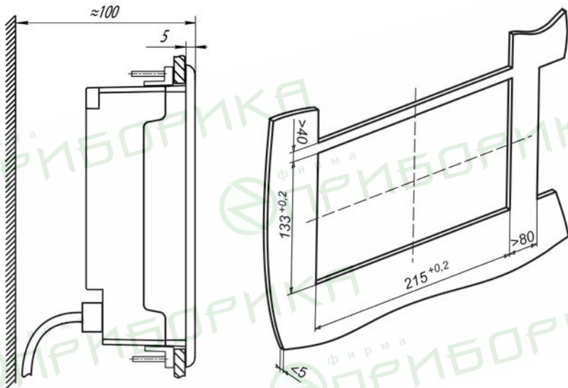
Рисунок А.2 – Установочные размеры
