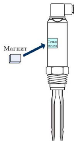
Рис. 5 Функция тестирования
