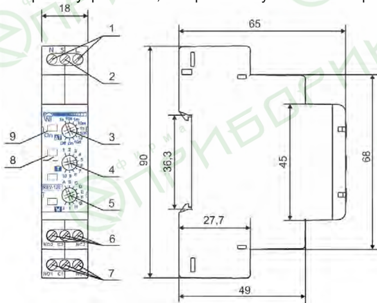
Рисунок 1 – Органы управления, габаритные и установочные размеры РЭВ–120
