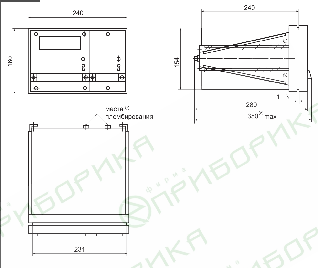
Габаритные и установочные размеры вторичного преобразователя РУ-ПТЗ.
