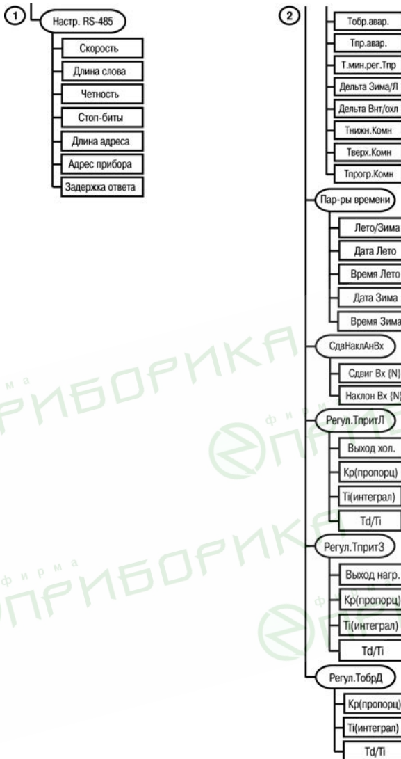
Рисунок И.1 – Главное меню прибора (продолжение)
