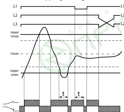
Диаграмма работы
