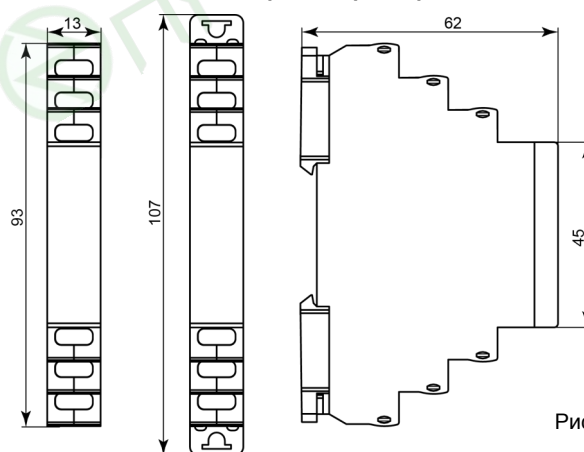
Габаритные размеры
