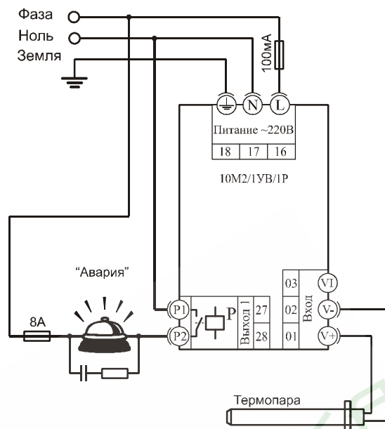
Схема 4. Типовая схема подключения прибора Термодат-10М2 для аварийной сигнализации о перегреве или снижении температуры. Вместо звонка может быть установлена лампочка.
