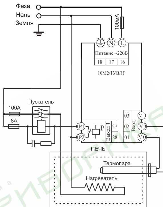
Схема 2. Типовая схема подключения прибора Термодат-10М2 для управления мощной печью. Реле Р включает электромагнитный пускатель. Пускатель включает нагрузку – однофазную или трёхфазную.
