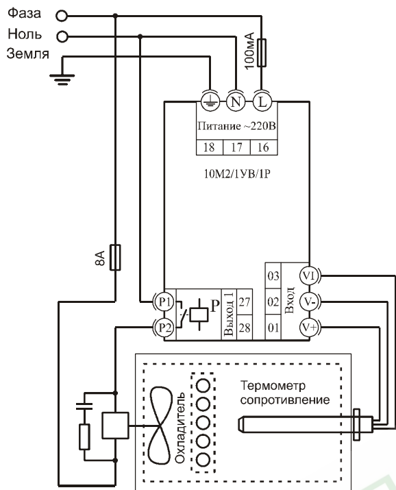
Схема 3. Типовая схема подключения прибора Термодат-10М2 для управления охлаждением
