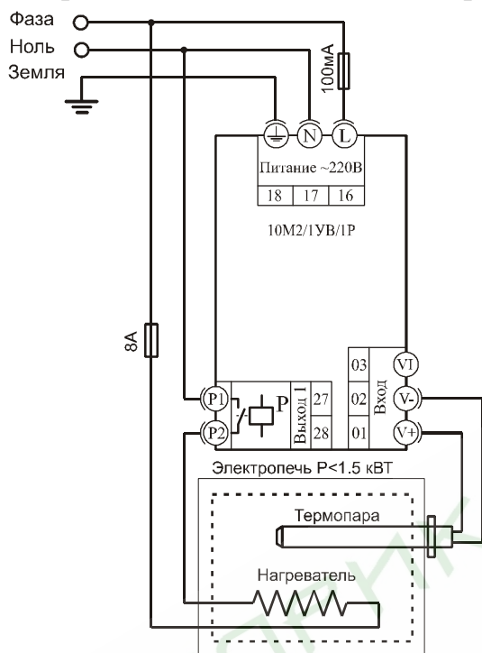
Схема 1. Типовая схема подключения прибора Термодат-10М2 для управления маломощной печью.
