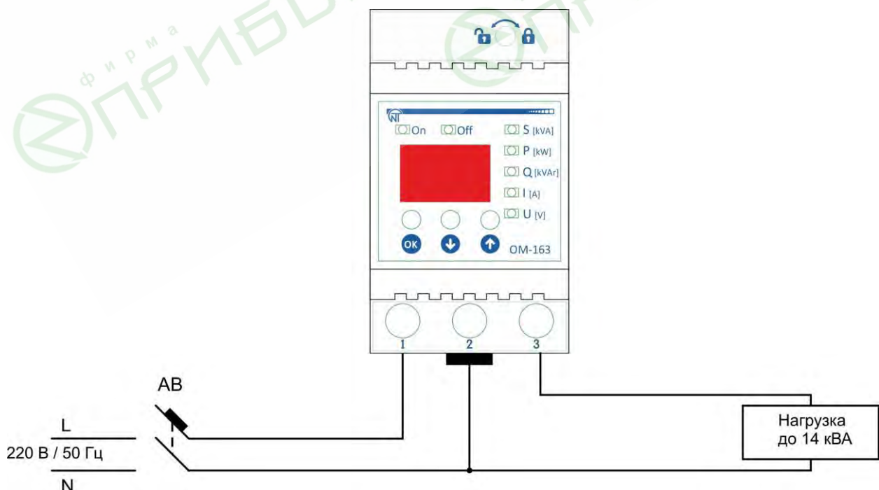
Рисунок 2 – Схема подключения изделия
