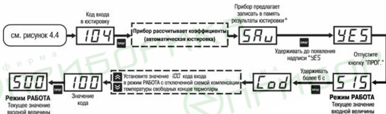
Рисунок Д.6 – Последовательность действий при юстировке схемы прибора с термопарой
