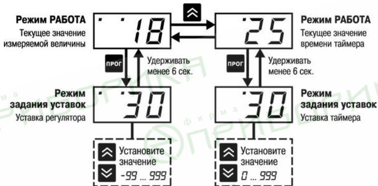
Рисунок 4.3 – Схема задания уставок регулятора и таймера
