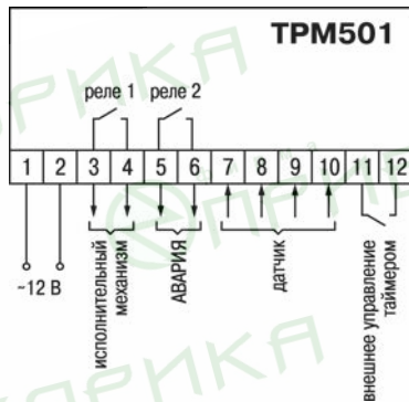
Рисунок Б.1 – Клеммник TPM 501
