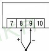
Рисунок 6.3 – Схема подключения термопары
