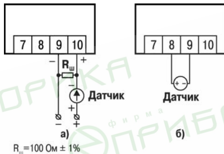
Рисунок 6.4 – Схема подключения датчиков с выходным сигналом тока (а) и напряжения (б)
