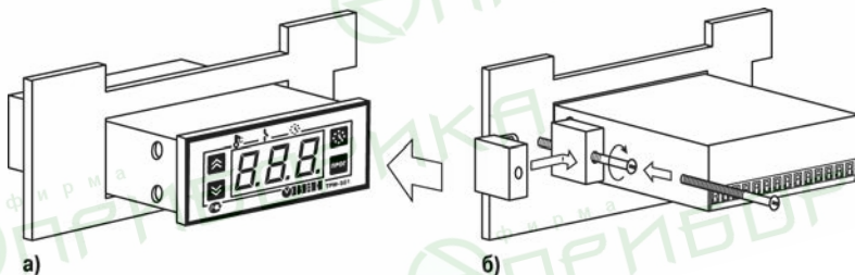
Рисунок 6.1 – Монтаж прибора
