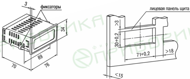
Рисунок А.1 – Габаритные и установочные размеры TRM501
