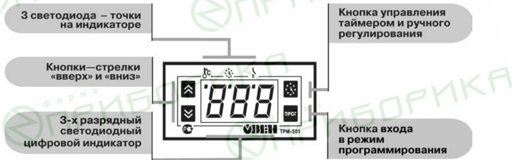
Рисунок 3.1 – Лицевая панель прибора
