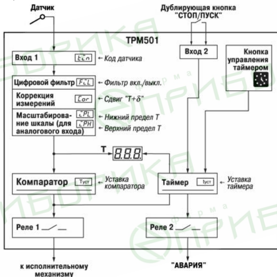
Рисунок 3.2 – Функциональная схема прибора
